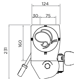
Loggia - Pose PLAFOND Sortie treuil à l'arrière
